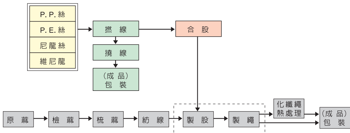
繩索製造流程圖
