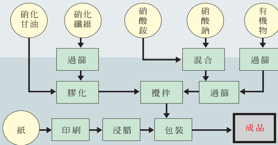
硝甘炸藥製造流程圖
