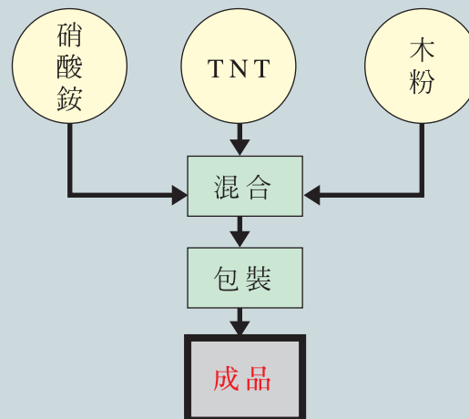
混合炸藥製作流程圖
