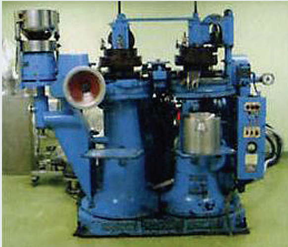
子母錠壓錠機。
