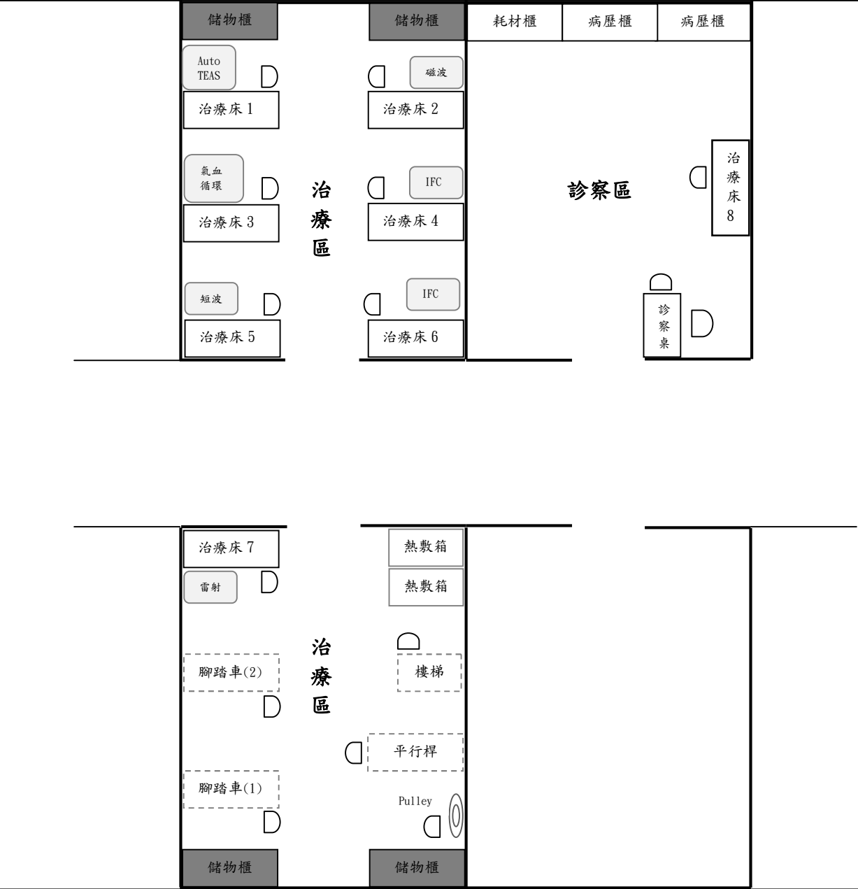
台北榮譽國民之家 復健診察及治療區平面配置示意圖 2 (NO SCALE)
