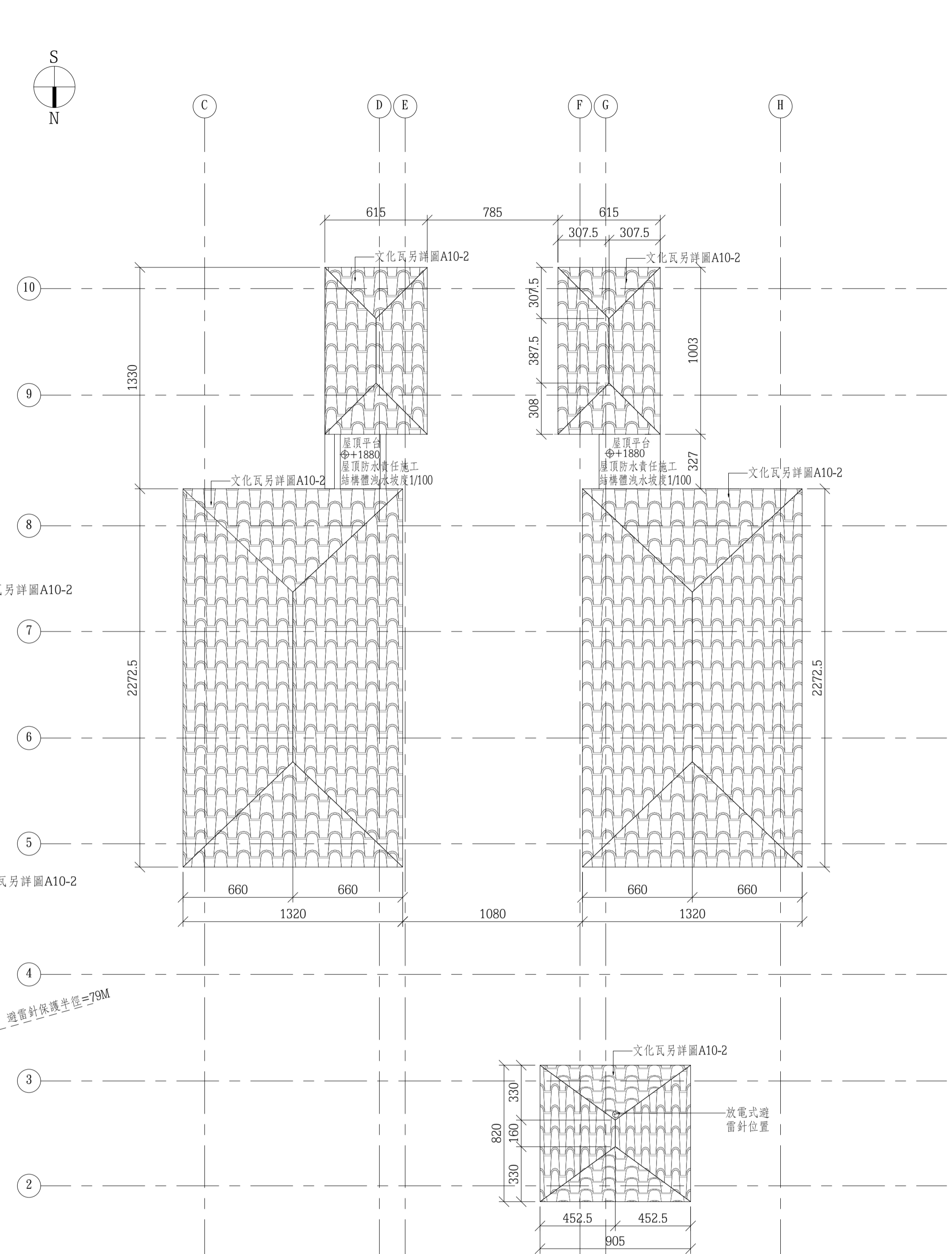
2 TFL 屋頂頂蓋平面圖 A1= 1:200 A3= 1:400
