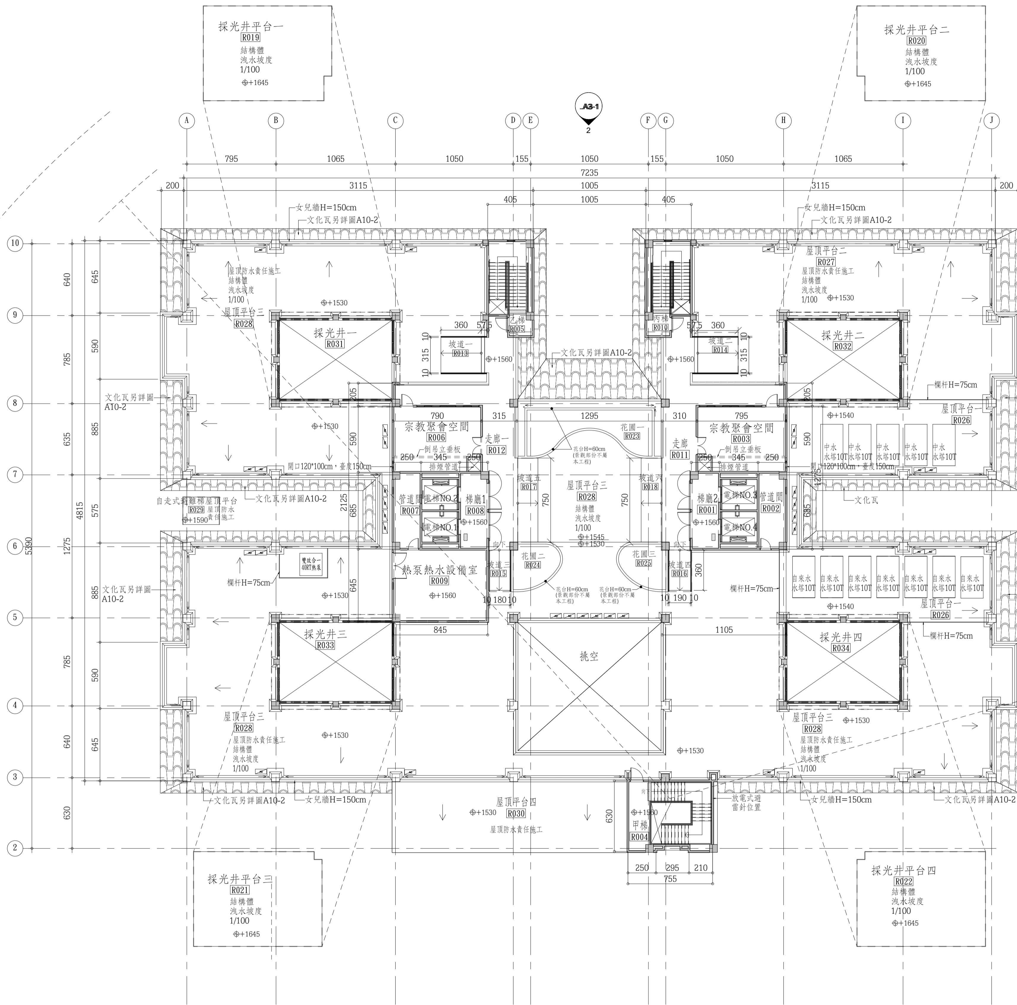
1 RFL 屋頂平面圖 A1= 1:200 A3= 1:400
